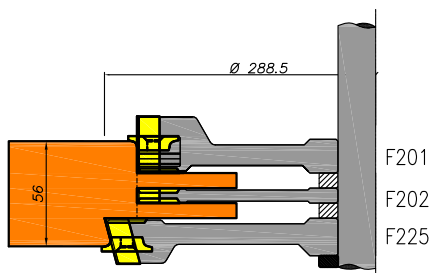
Stompe ramen stijl en bovendorpel verjongd
